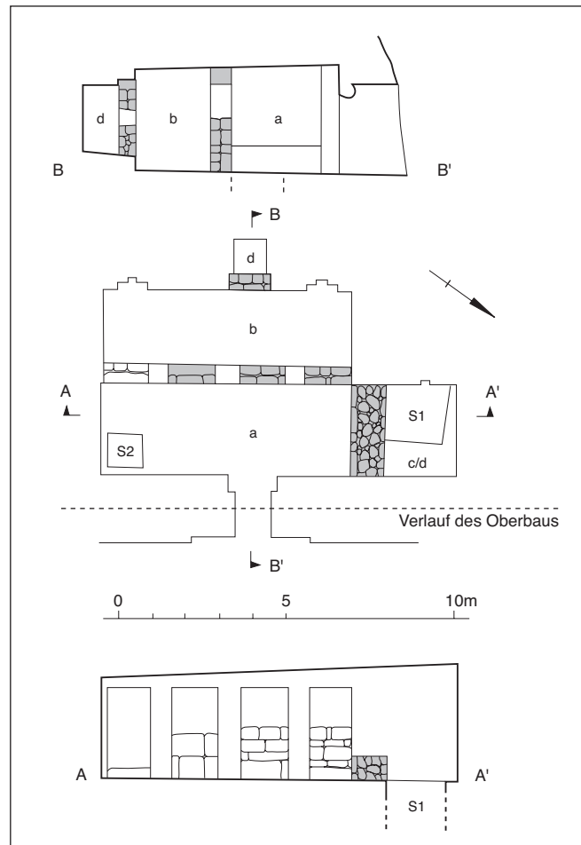
Abb. 124 Das Felsgrab MQ 1 des Chuenre
