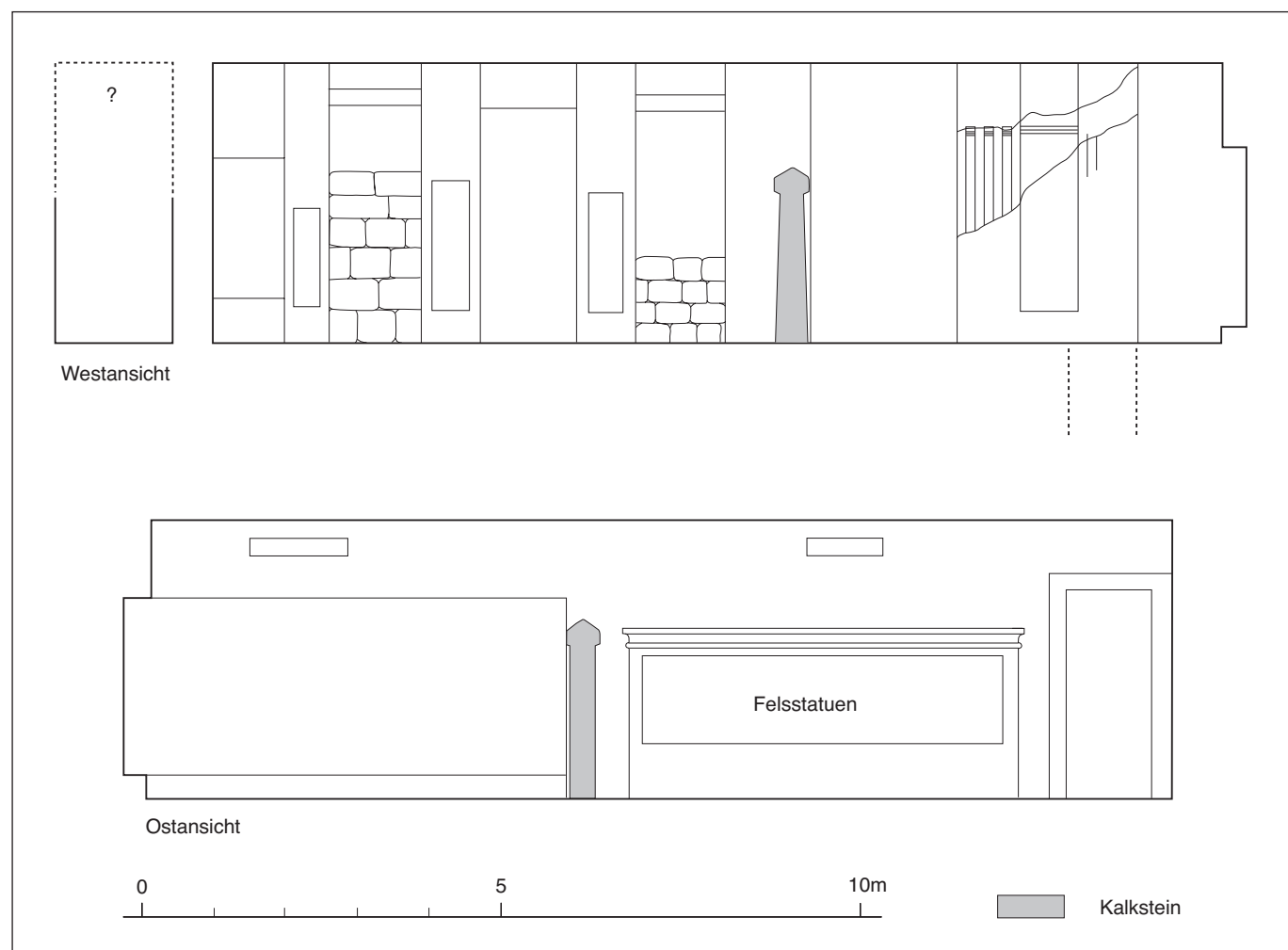
Abb. 107 Aufrisse des Felsgrabes LG 90
