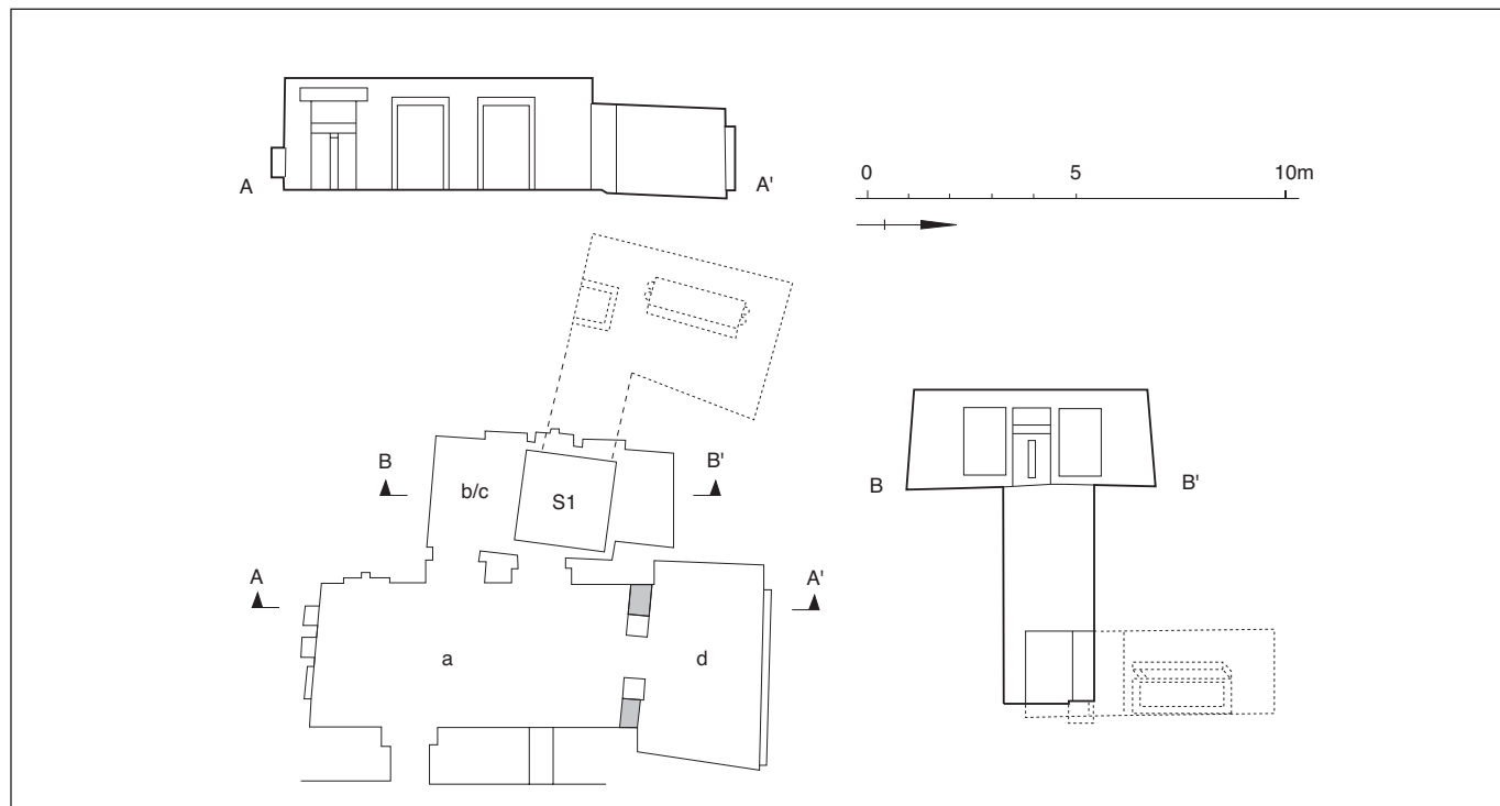
Abb. 86 Das Felsgrab der Königin Meresaneh III. G 7530 sub
