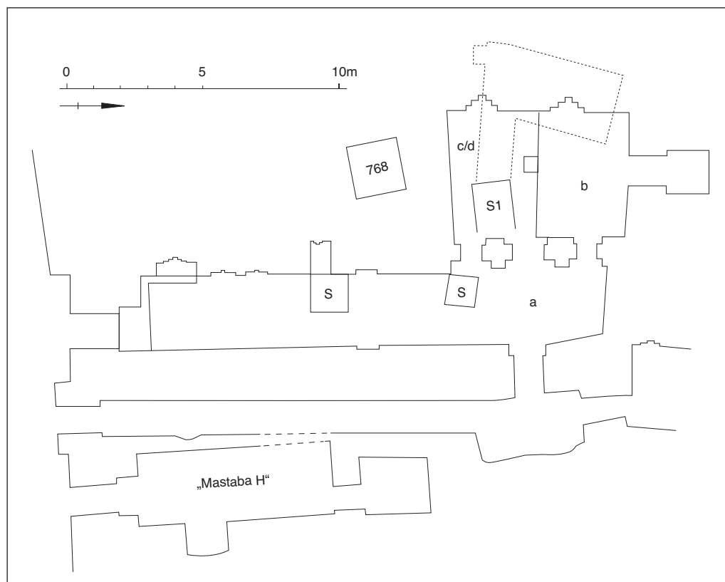
Abb. 116 Das Felsgrab der Königin Bunefer
