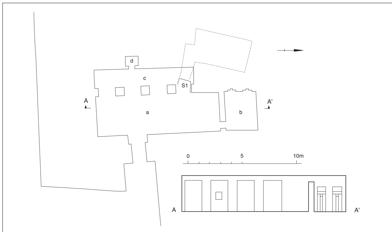
Abb. 121 Rekonstruktion des möglichen ursprünglich geplanten Bauzustandes des Hemetre-Grabes im Central Field
