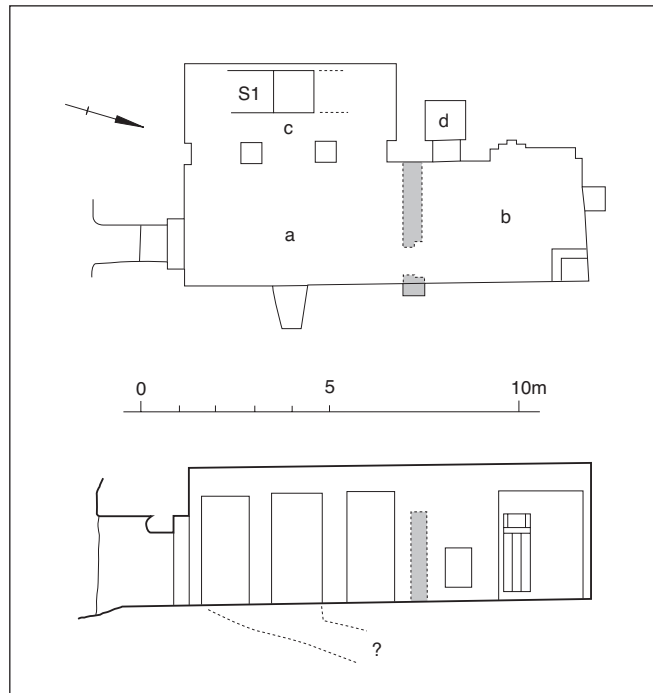
Abb. 98 Das Felsgrab LG 88 der Per[senet]
