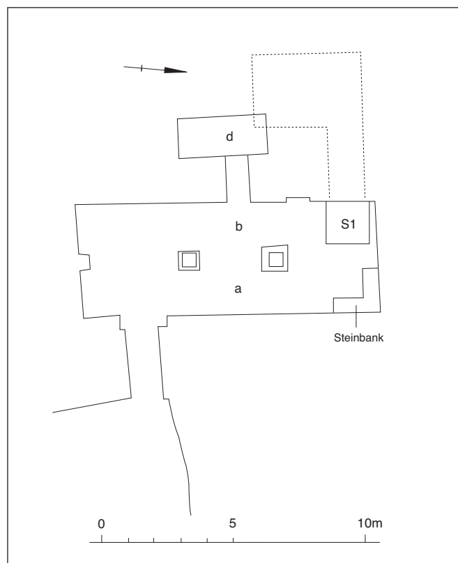
Abb. 103 Das Felsgrab des Niuserre
